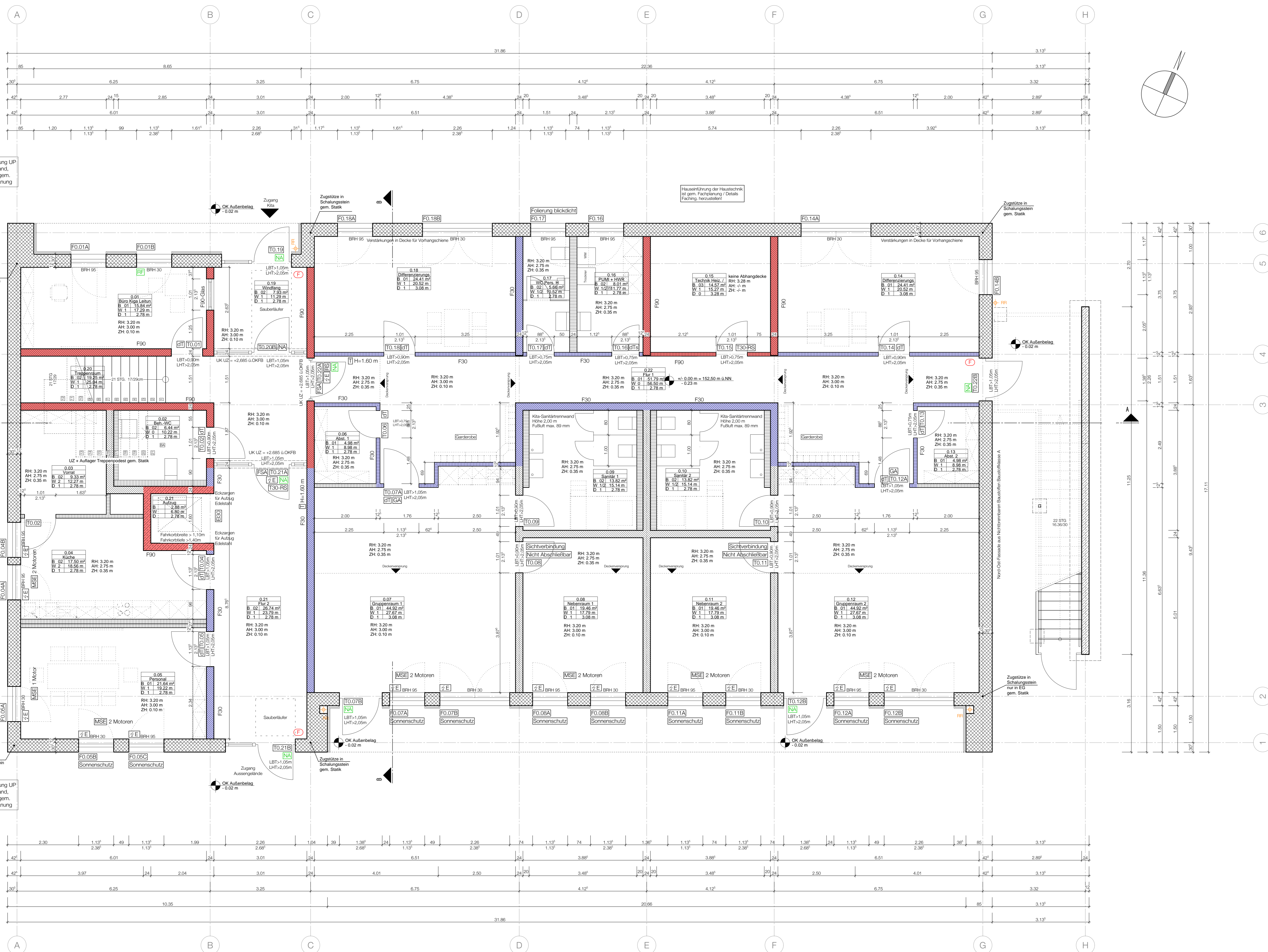
Grundriss ERDGESCHOSS
